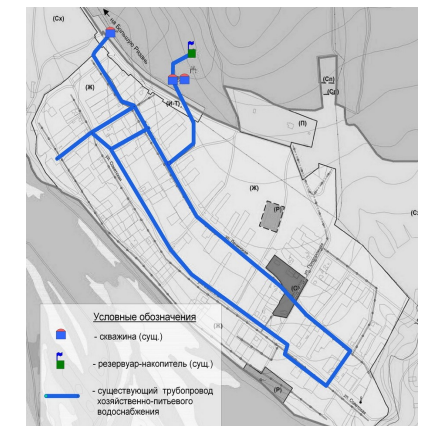
Рисунок 2.4.9.2 – Существующая схема централизованного водоснабжения
