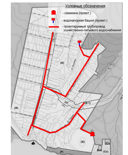
Рисунок 2.4.9.4 – Перспективная схема развития централизованного водоснабжения с.п. Малая Рязань
