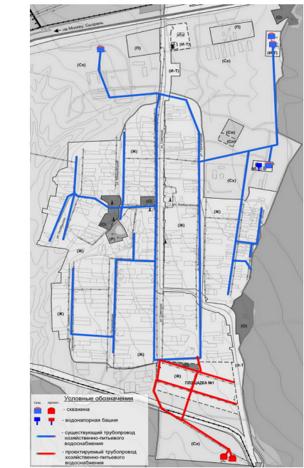
Рисунок 2.4.9.1 – Существующая и перспективная схема развития централизованного водоснабжения с.п. Большая Рязань
